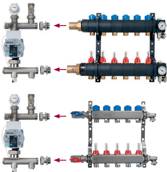
Bij een RVS verdeler tot 8-groepen moeten de kogelkranen eerst verwijderd worden.
